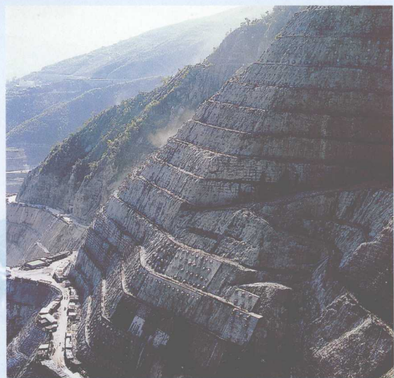
云南小湾水电站高边坡锚固工程
