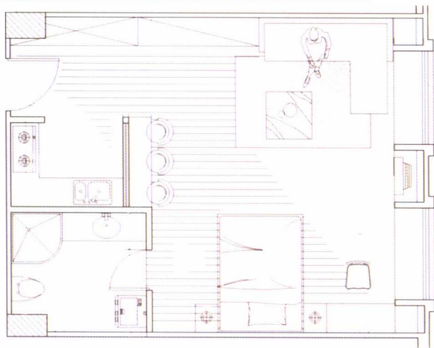
平面图
