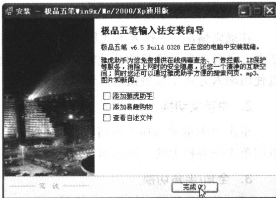
图 1-5 “完成”界面
