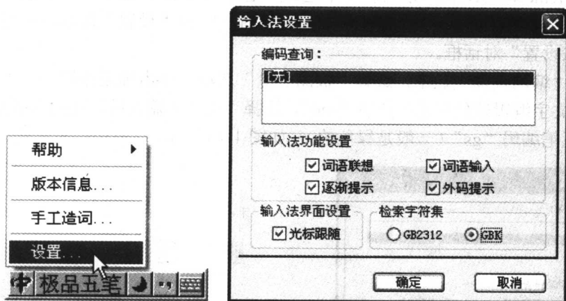
图 1-14 输入法设置
