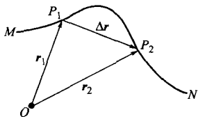
图 1-2 位移矢量
