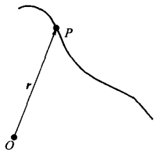
图 1-1 位置矢量
