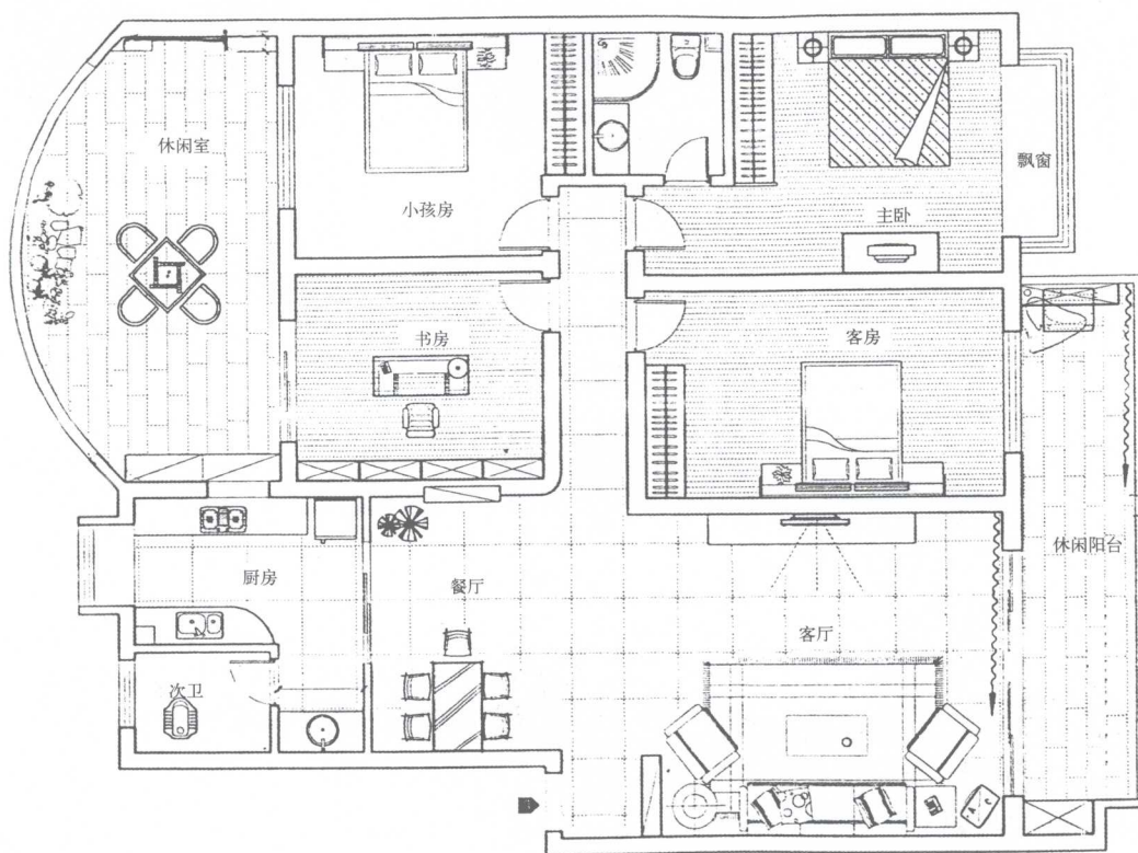
平面布置图
