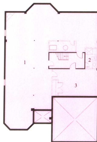
地下室
