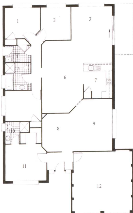
首层 (方案A)
