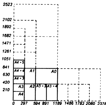
图 1-1 图纸幅面尺寸
