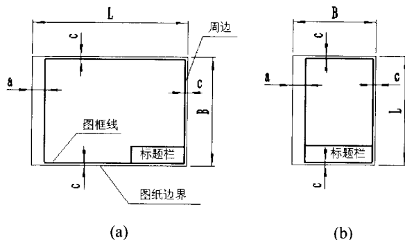
图 1-2 留有装订边图样的图框格式
