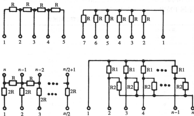
图 1-4 排电阻内部电路
