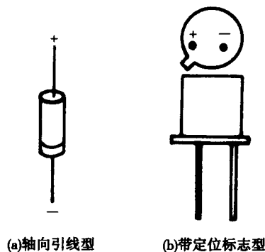
图 1-10 二极管极性识别示意图
