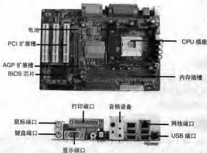
图 1-2 微型计算机主板
