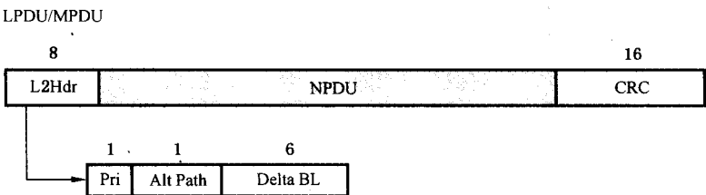
图 6 MPDU/LPDU 格式
