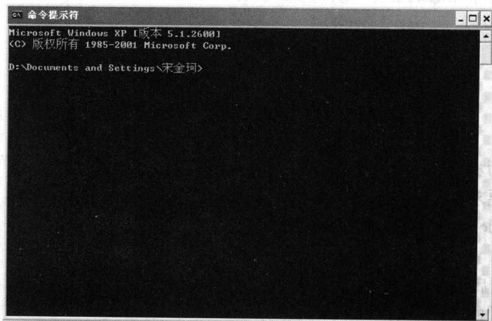
图 1-4 DOS 界面
