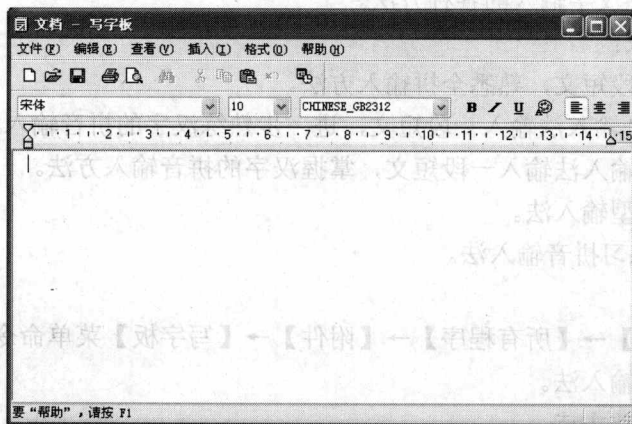
图 1-6 写字板
