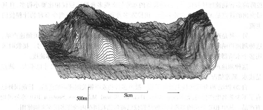
图 1.3 多波束回波测深仪测得的海底三维地形
