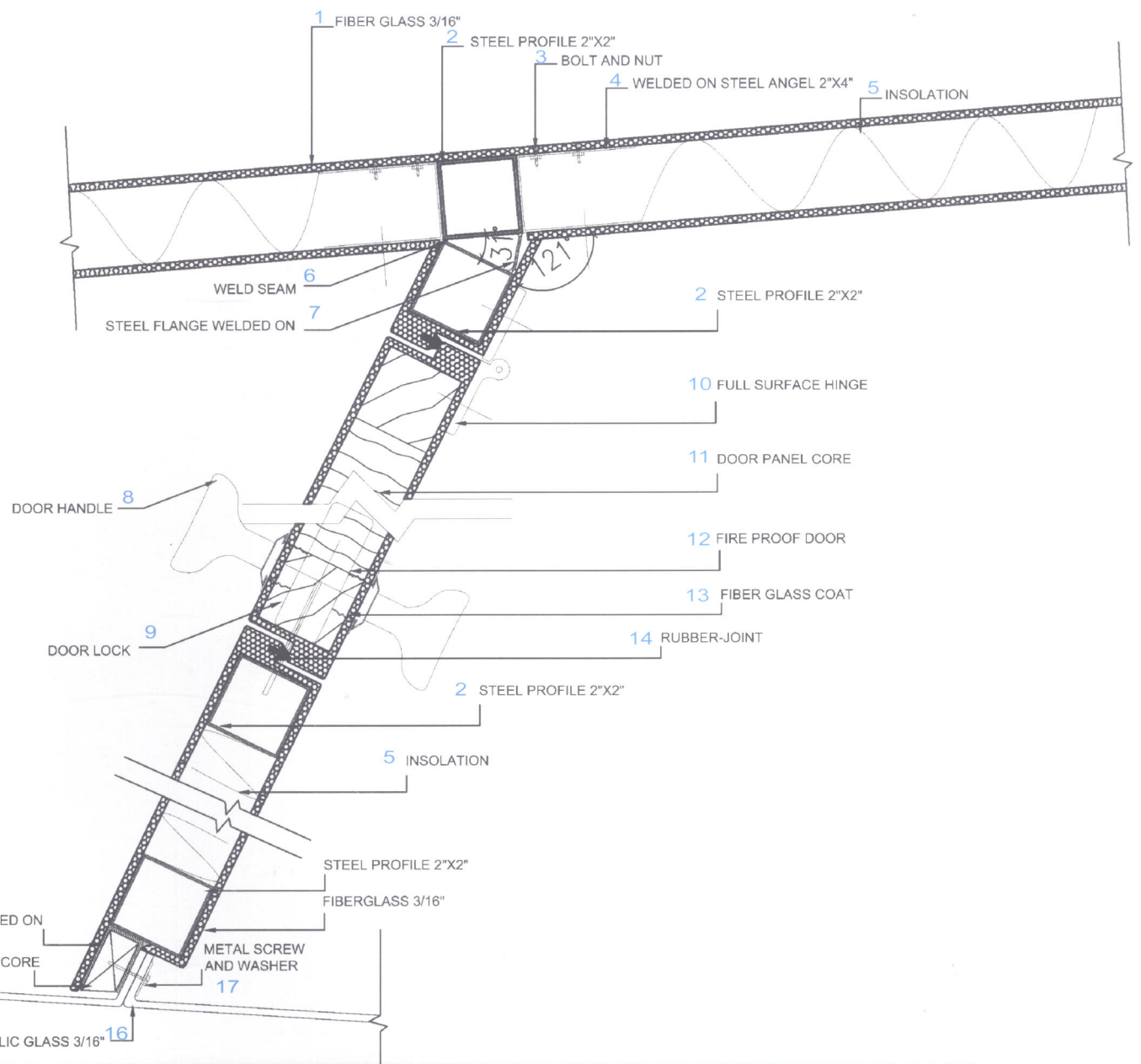
门内详图 Door inside detail
