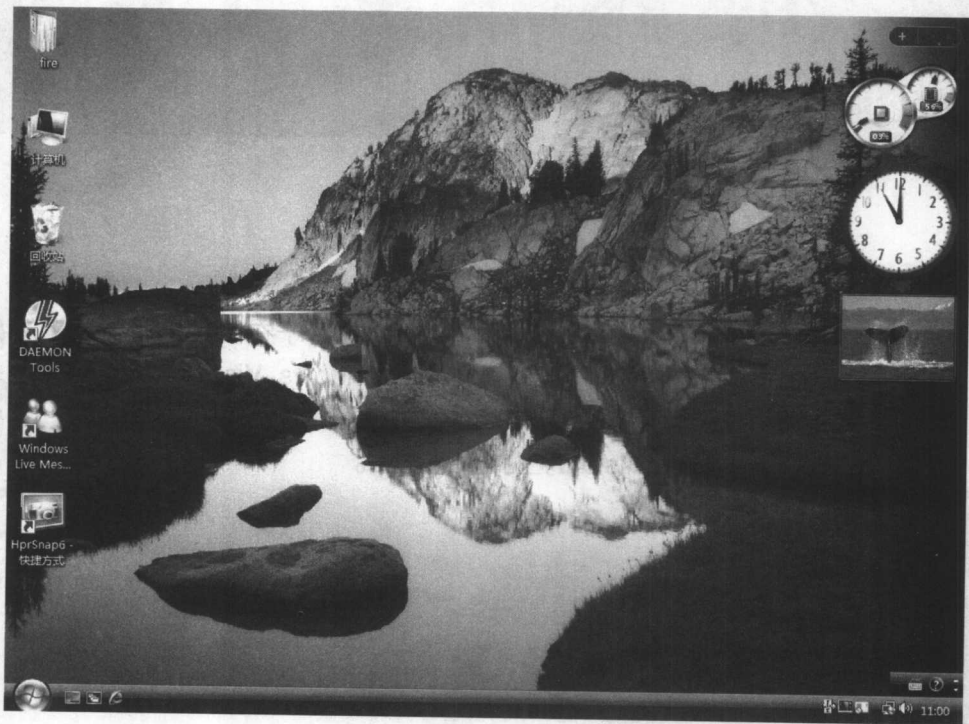
图1-1 Windows边栏
