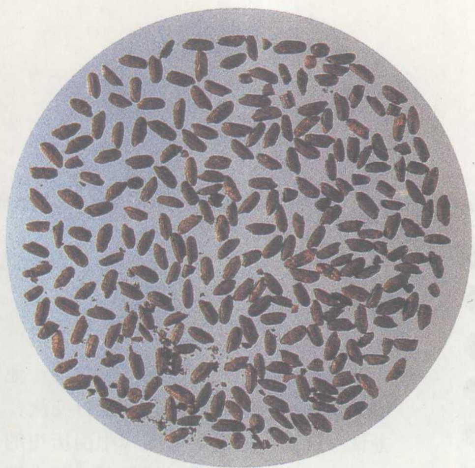
炭化水稻粒
