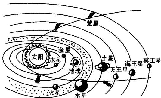
图 1.1 太阳系、地球在太阳系中的位置
