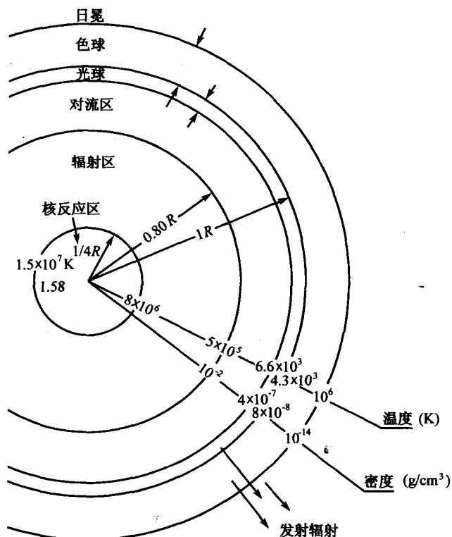
图 1.2 太阳结构示意图
