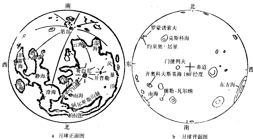
图 1.3 月球表面形状分布
