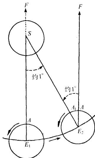
图1.4 恒星日与太阳日示意图
