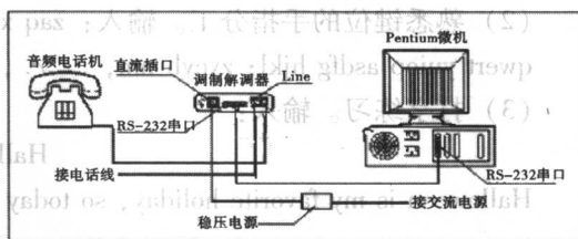
图 1-4 拨号上网硬件连接方法
