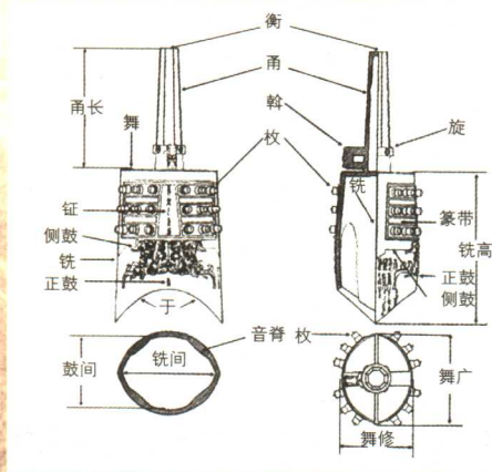
战国曾侯乙编钟结构图
