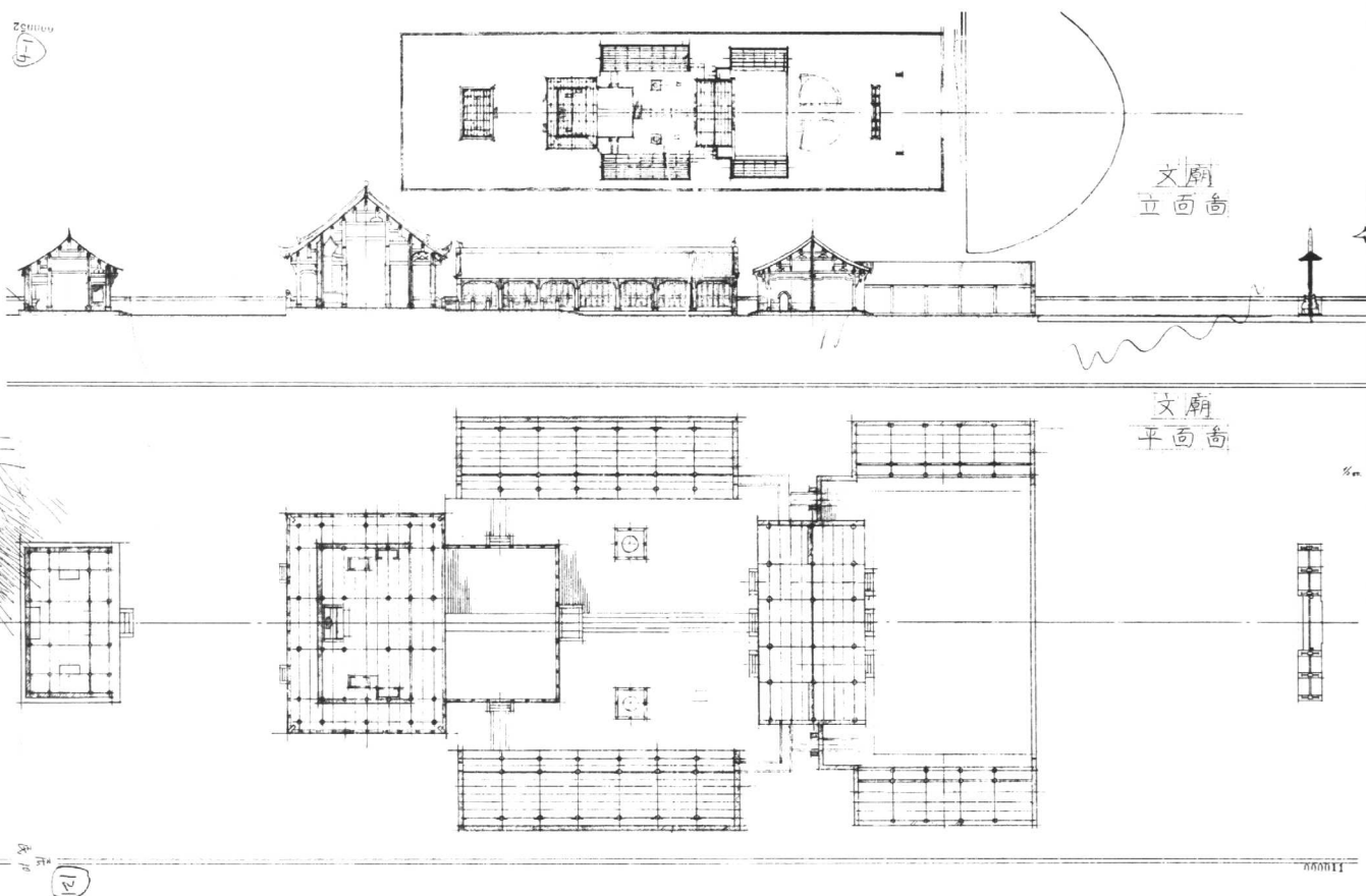
昆明文庙立面、平面
