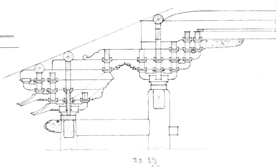
真庆观大殿柱头科斗拱
