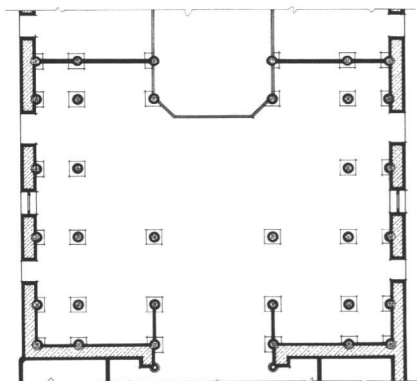
昆明城隍庙大殿 (改为大众影院)
