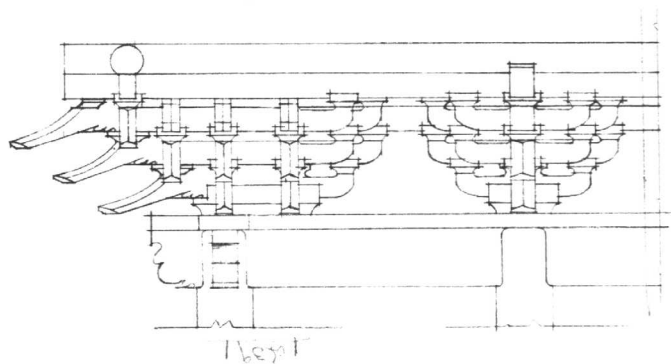
真庆观大殿柱头科斗拱
