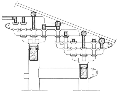
昆明城隍庙大殿斗拱
