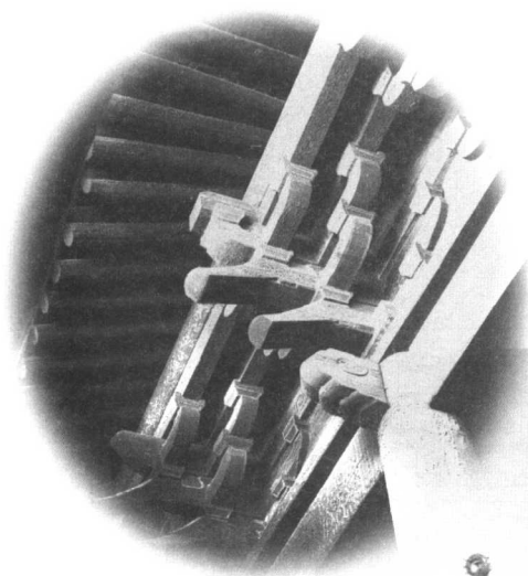
真庆观大殿 外檐斗拱
