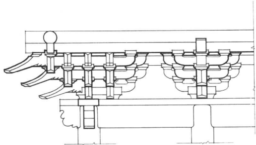
真庆观大殿角科斗拱
