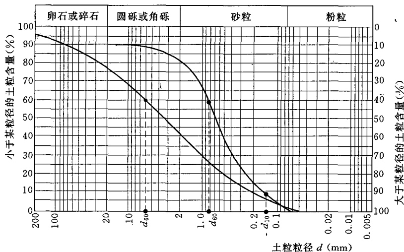
图 1-5 颗粒级配曲线
