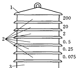
图 1-4 标准筛（单位：mm） 1—筛盖；2—筛盘；3—底盘
