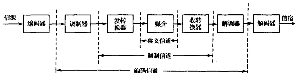
图 2.1 信道的分类
