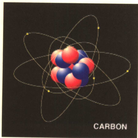
碳原子模型
