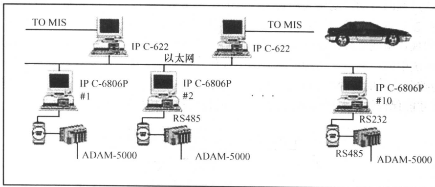
图 1.5 汽车出厂检验原理
