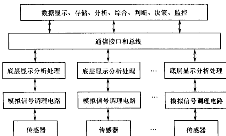
图 1.2 检测系统的一般构成框图
