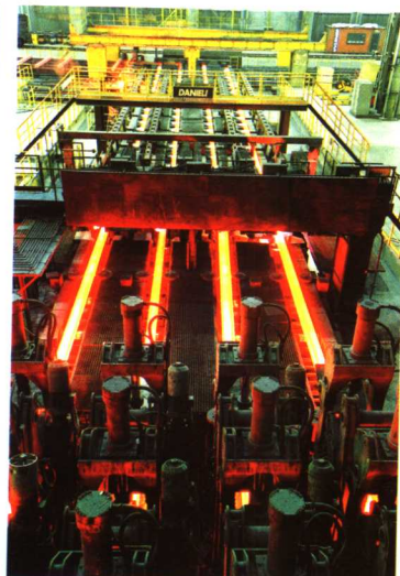
四机四流弧形方坯连铸机
