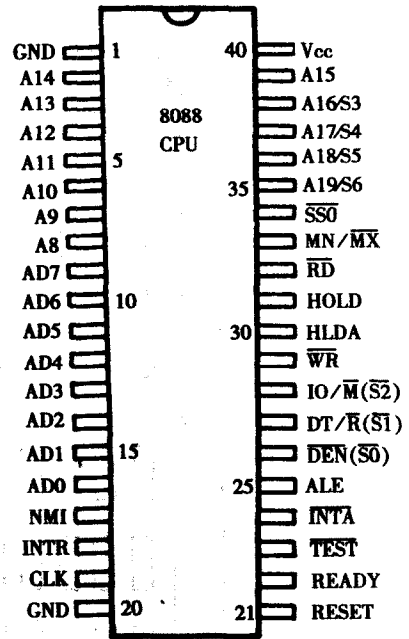
图 1.4 8088 CPU 引脚排列
