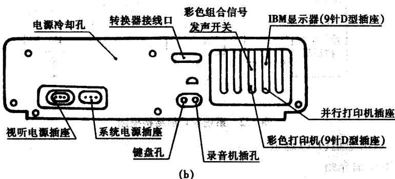
图 1.1 IBM PC/XT 微机系统装配示意图
