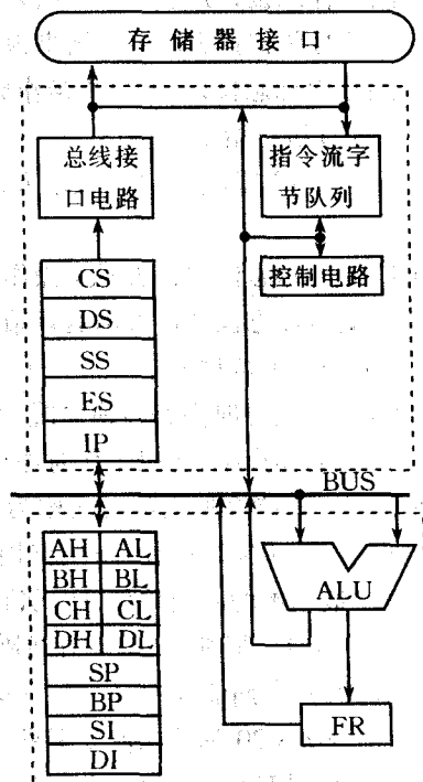
图 1.5 8088CPU 内部结构
