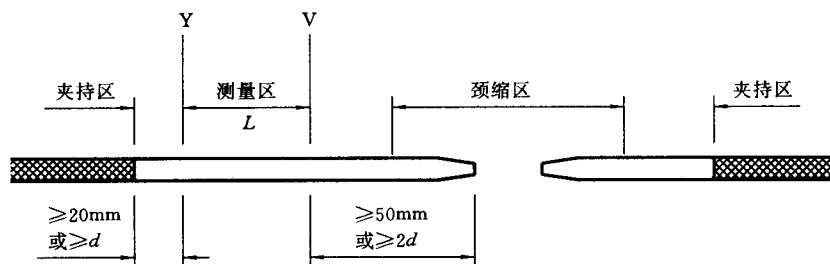
图 A1 断裂后的测量
