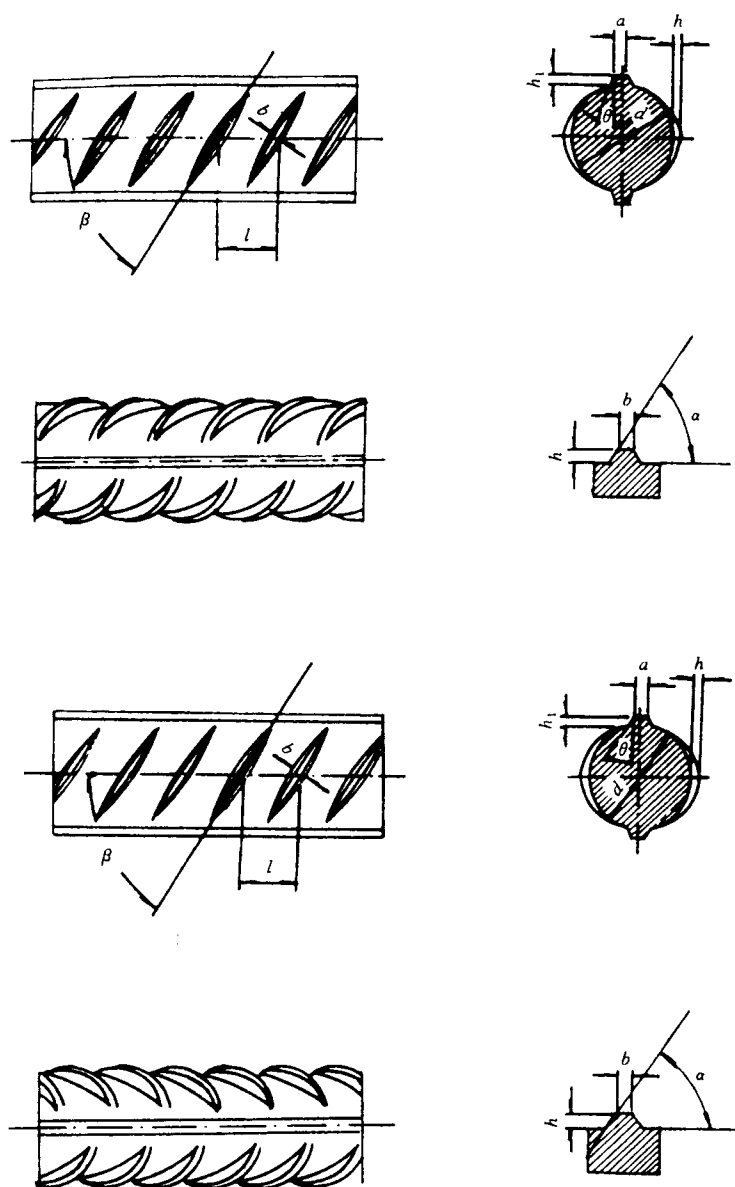
d —钢筋内径； a —横肋斜角； h —横肋高度； \beta —横肋与轴线夹角； h_1 —纵肋高度； \theta —纵肋斜角； \alpha —纵肋顶宽； l —横肋间距； b —横肋顶宽
