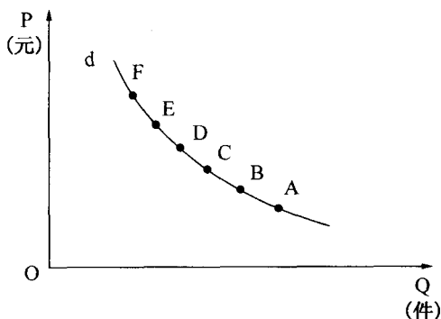
图 1-1 需求曲线
