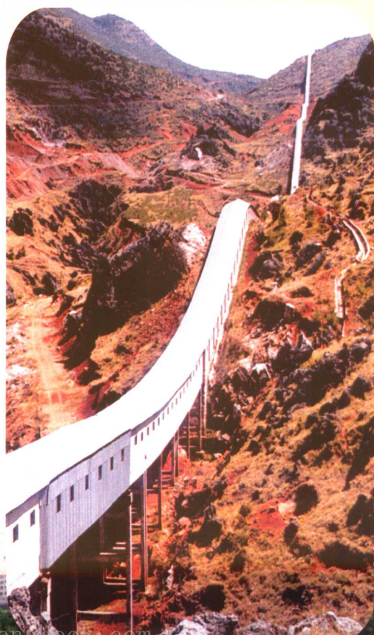
晋宁磷矿皮带运输线
