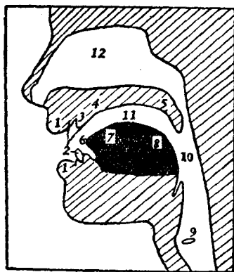
语音器官图
