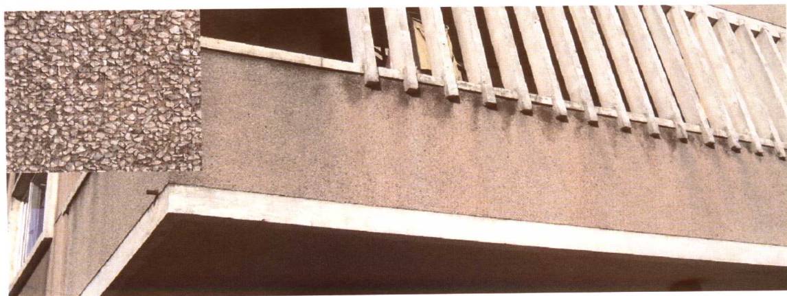
图 2-19 石粒类装饰抹灰(干粘石)
