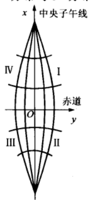
图 1-8 高斯平面直角坐标系的建立
