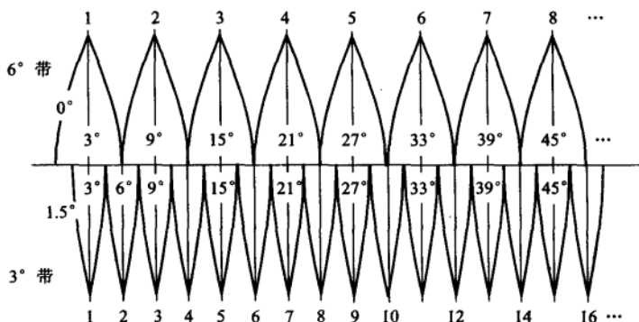
图 1-10 6° 与 3° 带的关系
