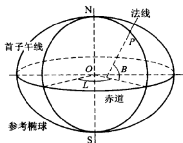
图 1-6 大地坐标系
