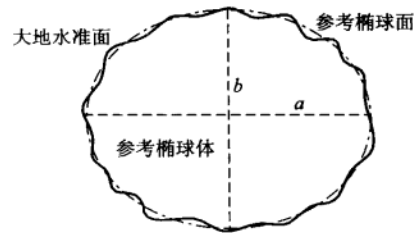
图 1-3 参考椭球面
