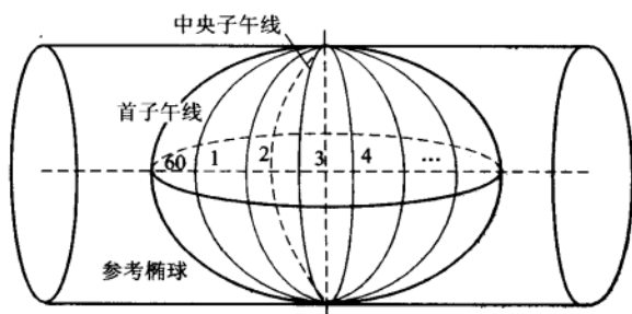
图 1-7 高斯投影示意
