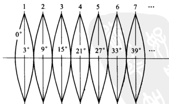
图 1-9 6^\circ 投影带
