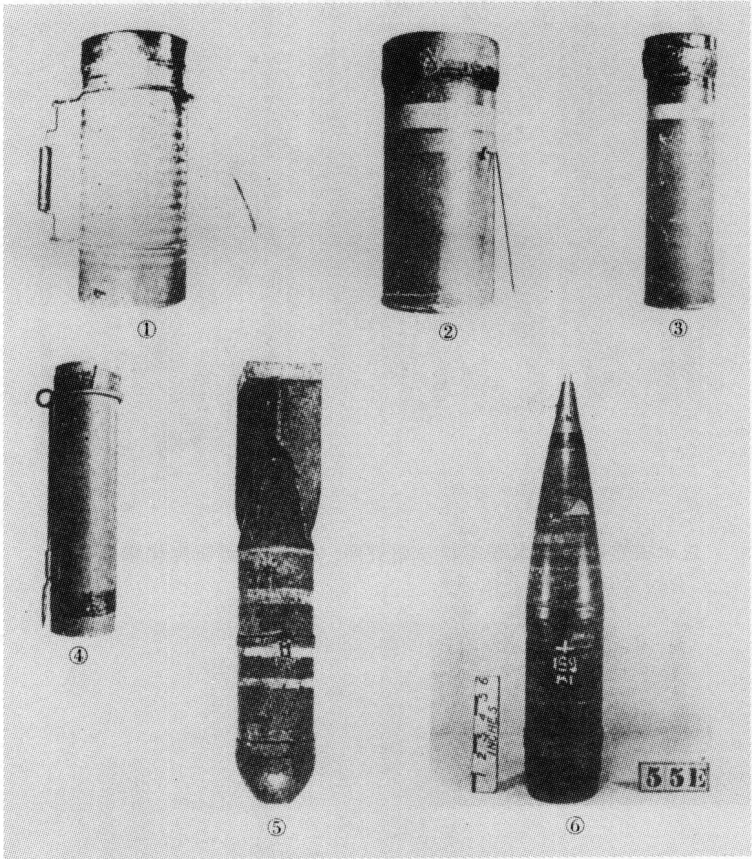
日军装备的化学弹药
