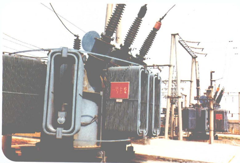
运行中的110千伏 变电站主变压器
