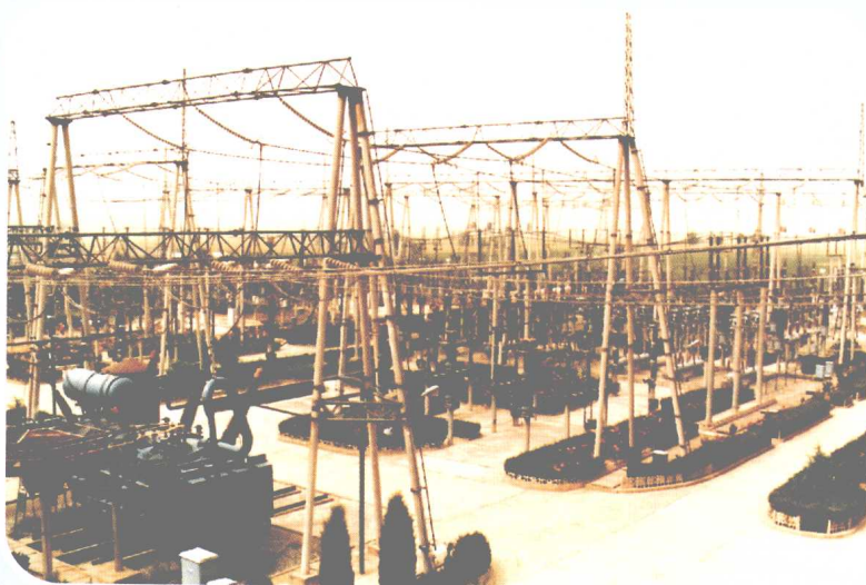
330千伏庄头变电站室外设备
