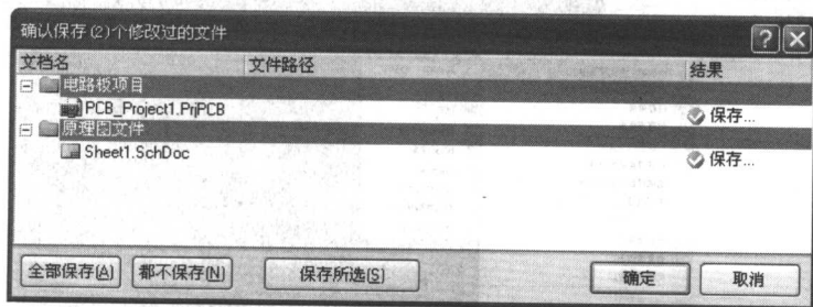
图 1-12 保存确认
