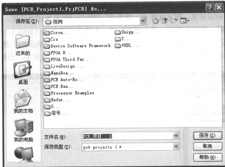
图 1-9 另存项目
