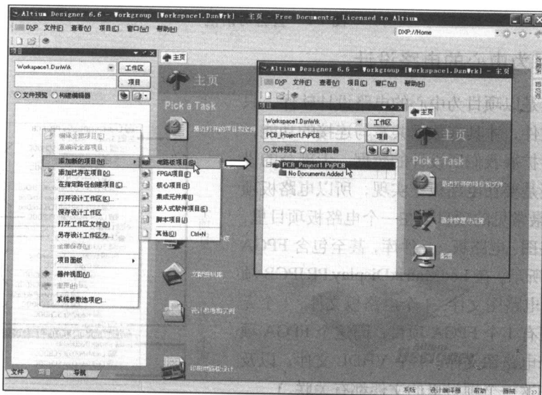
图 1-8 打开新项目
