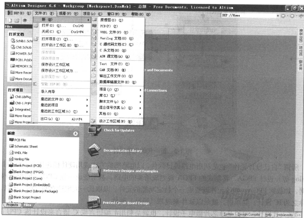
图 1-3 Designer 界面
