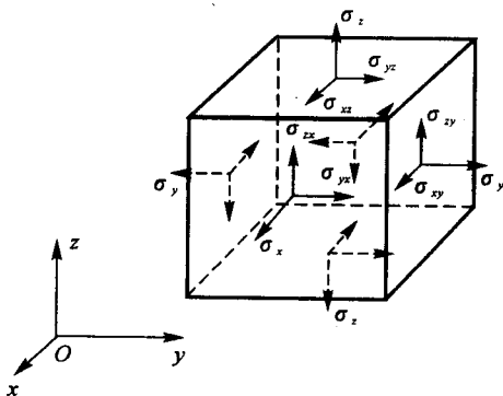
图 1-2 弹性体应力状态
