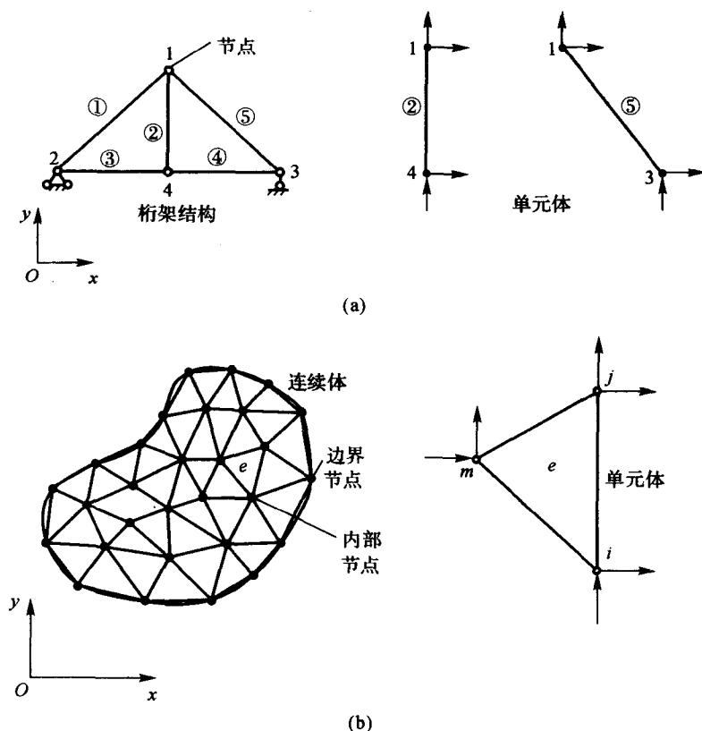
图 1-1 结构及连续体的离散化
