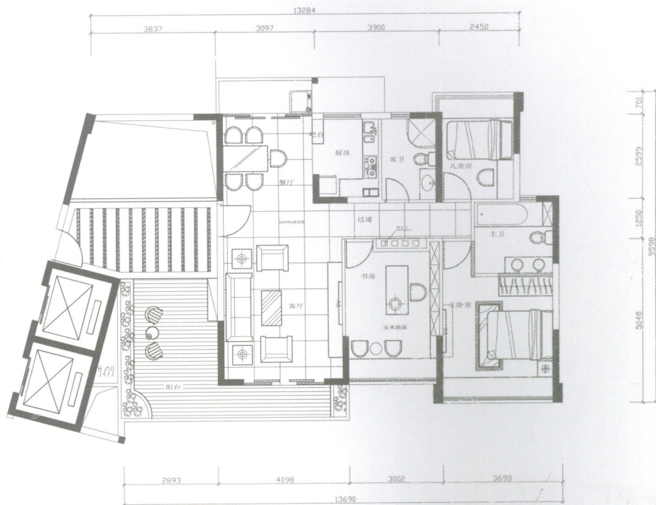
9#3楼B套平面布置图
