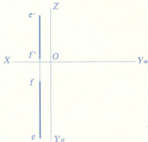
第三投影法
