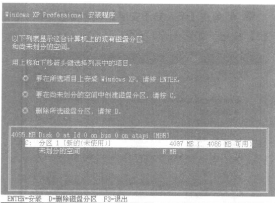
图 1-16 分区结束
