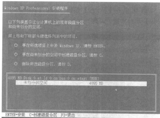
图 1-14 分区
