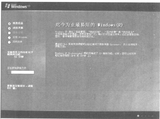
图 1-11 准备安装
