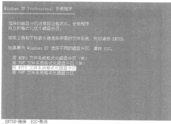
图 1-17 格式化磁盘
