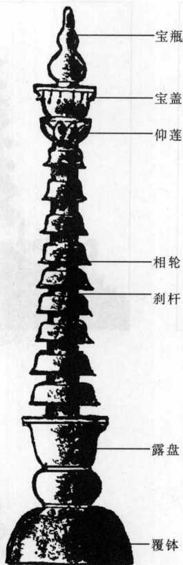
图7 广州六榕寺花塔的金属塔刹
