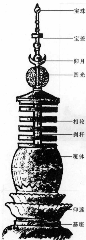
图6 山西应县佛宫寺释迦塔的金属塔刹(辽)
