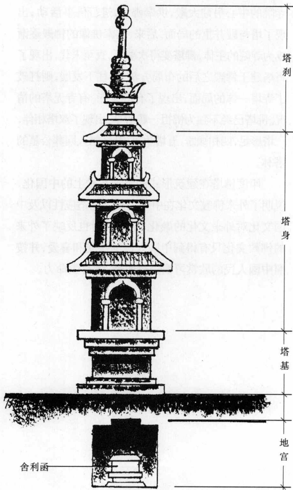
图2 塔的结构示意图
