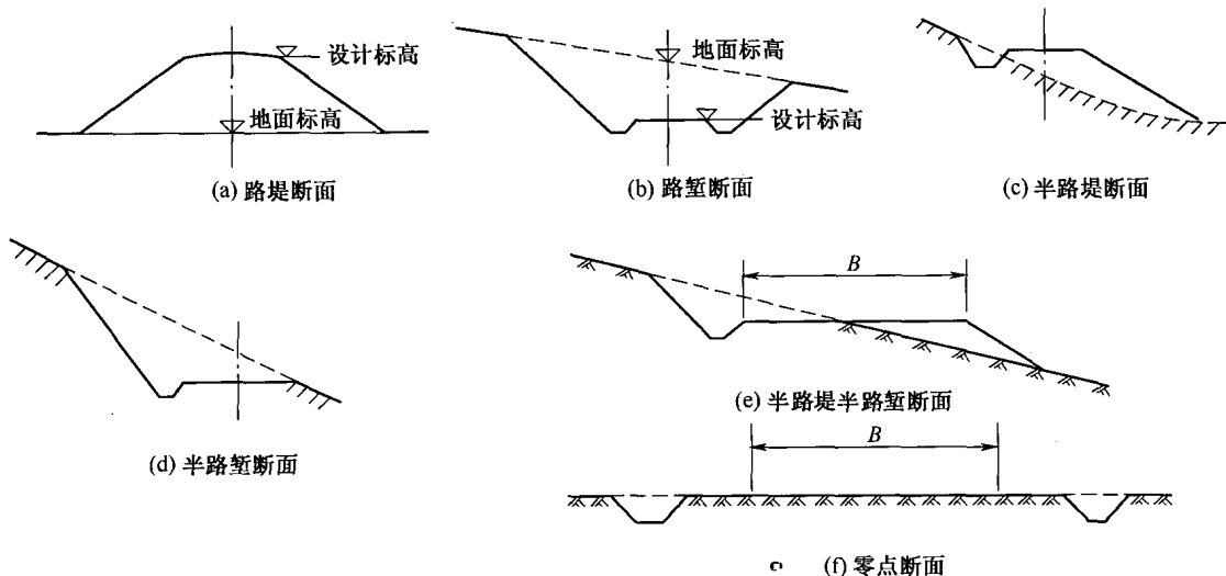
图 1-1 路基横断面形式
