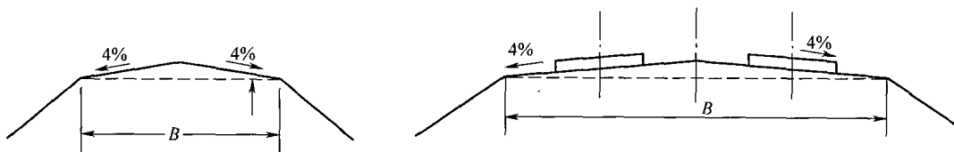
图 1-5 单、双线基路拱图 B—路基宽度
