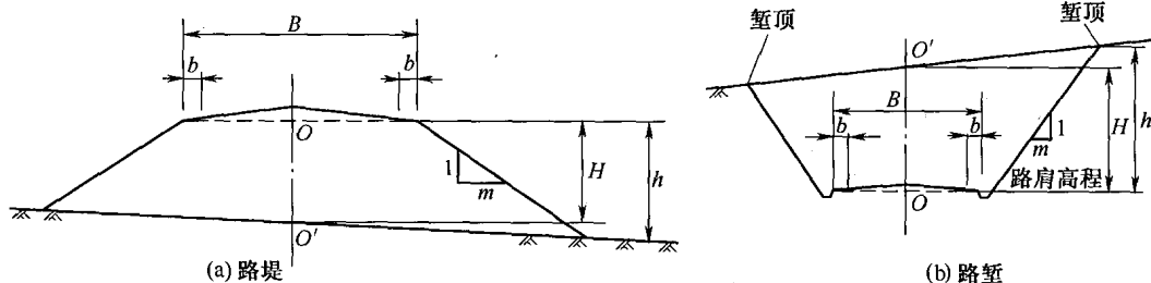
图 1-2 路基本体
