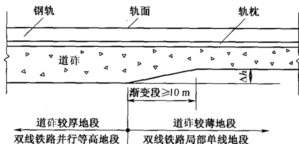
图 1-6 岩石、渗水土路基与非渗水土路基的衔接
