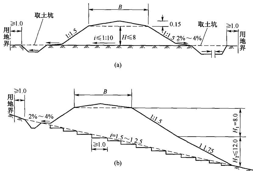
图 1-3 路堤标准横断面(单位:m)
