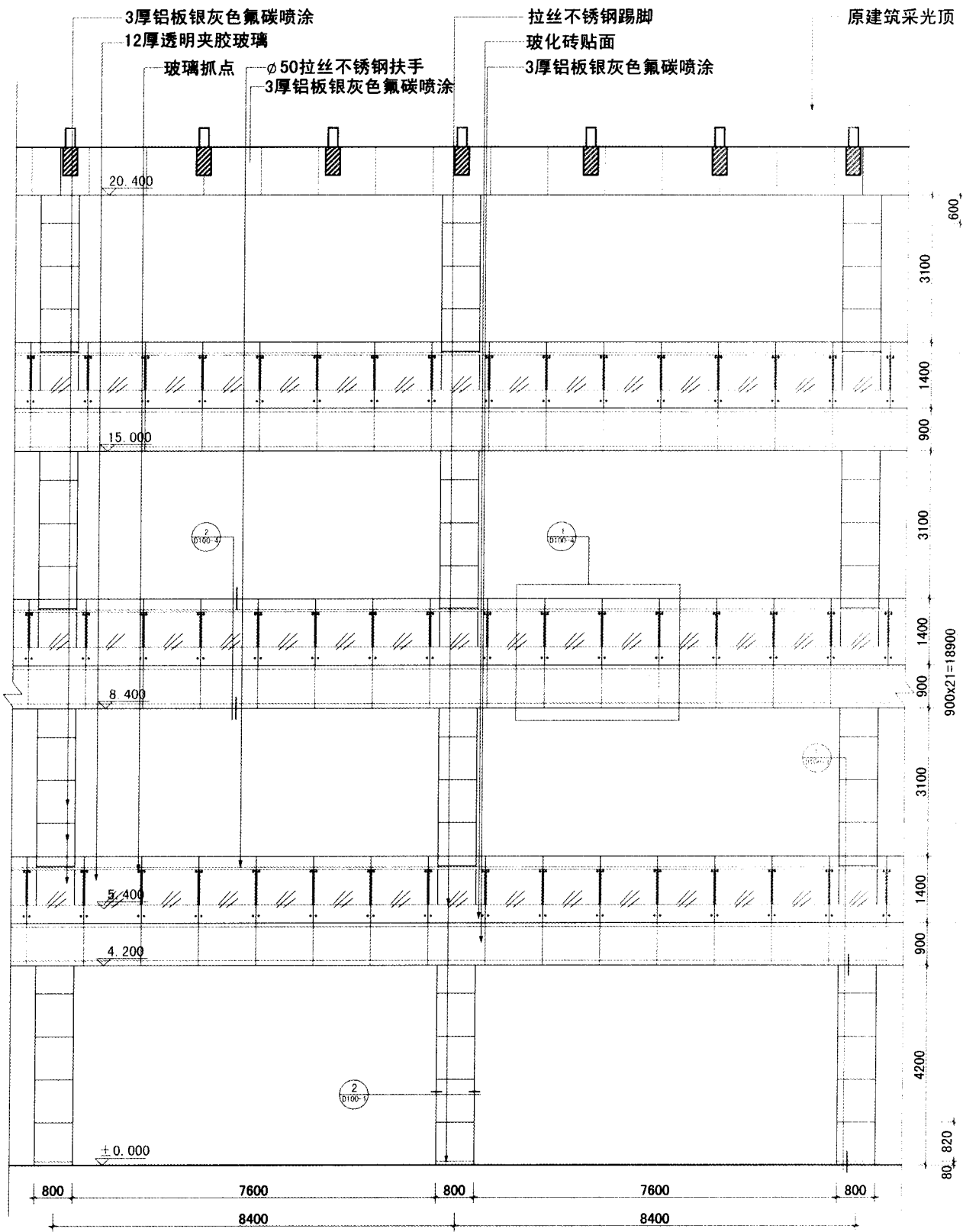
1 中厅立面展开图 E100-4
