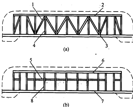
图 2-3 侧壁承载式车体的侧壁结构示意图
