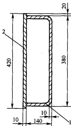
图 2-7 侧梁
