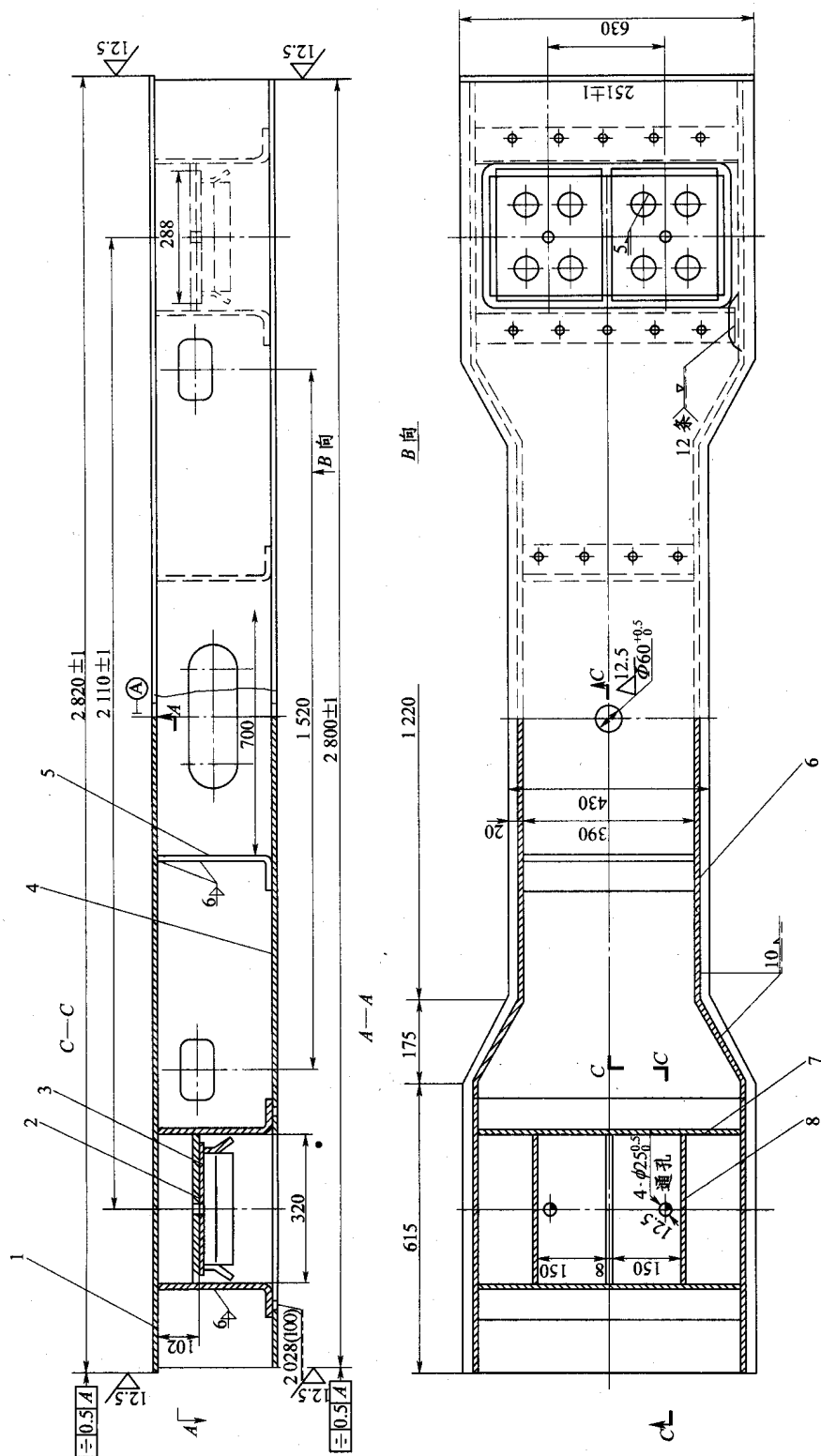
图 2-8 枕梁
