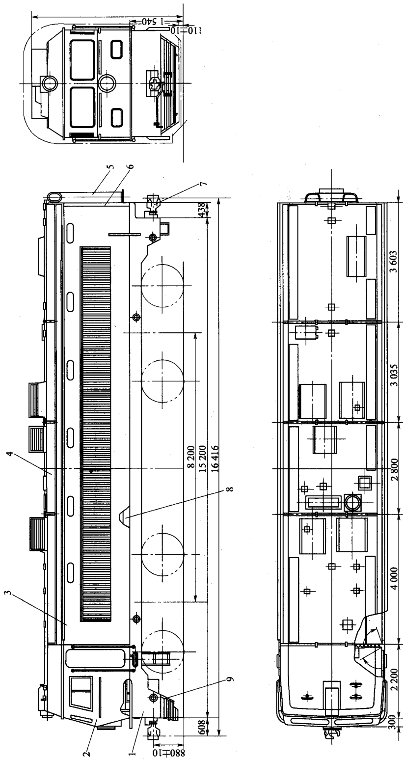
图 2-5 SS 4 改型电力机车车体总图 1—底架;2—司机室;3—侧墙;4—车顶盖;5—悬挂装置;6—后端墙;7—牵引缓冲装置;8—台架;9—排障器
