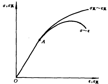
图 1.4 真应力—真应变曲线
