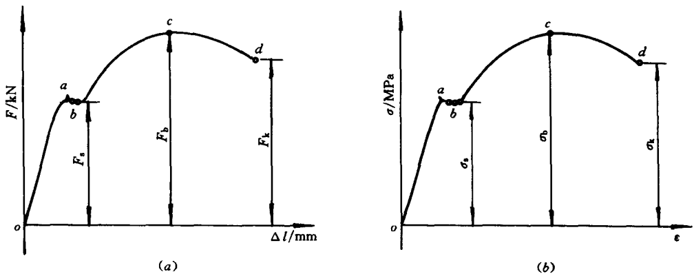
图 1.2 低碳钢的拉伸图(a)和应力—应变曲线(b)
