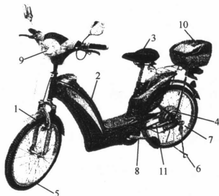
1—前叉；2—电池盒；3—鞍座；4—电机；5—内外胎； 6—支架；7—轮圈；8—链条曲柄；9—大灯； 10—后货箱；11—链条
