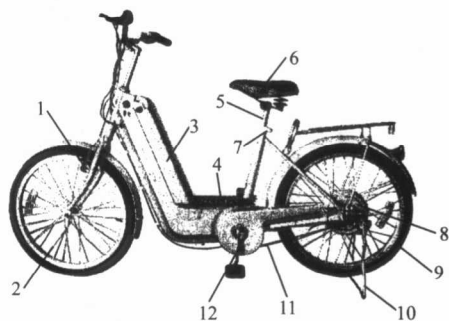
1—前叉；2—轮圈；3—电池盒；4—控制器（盖板内）； 5—鞍管；6—鞍座；7—鞍管螺栓；8—电机；9—内外胎； 10—支架；11—链条；12—链轮曲柄
