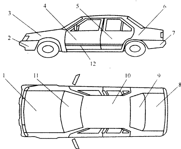
图 1-3 轿车车身各部位示意图
