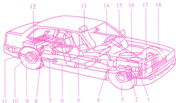
图 1-2 车身构造示意图
