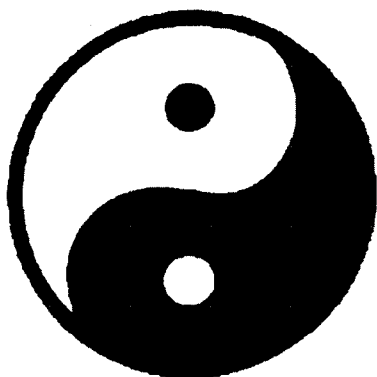
图3 太极图中的圆
