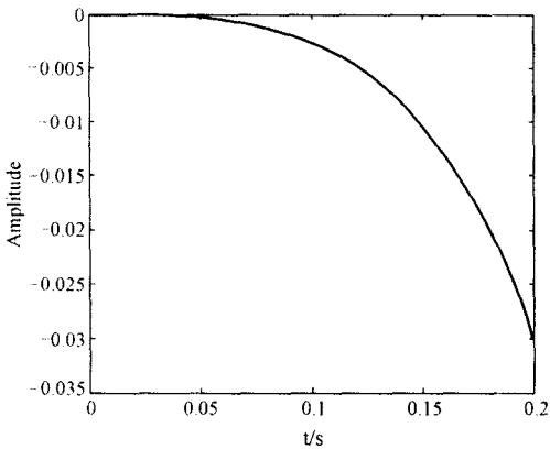
图 1-1 某控制系统的单位阶跃响应曲线
