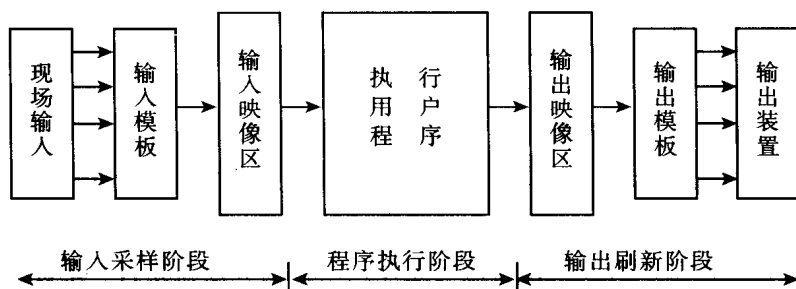
图 1-2 PLC 的工作过程
