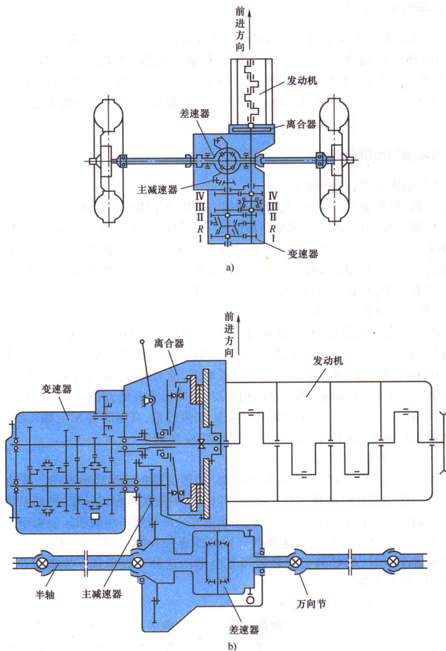
图 1-3 发动机前置、前轮驱动的轿车传动系示意图 a) 发动机纵向布置; b) 发动机横向布置
