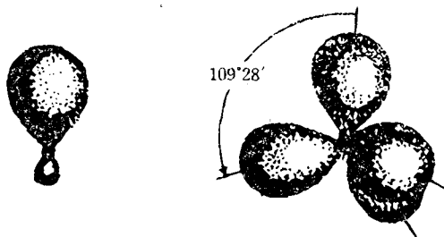
图 1-1 sp^3 杂化轨道
