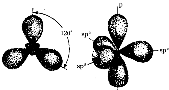
图 1-3 sp^2 杂化
